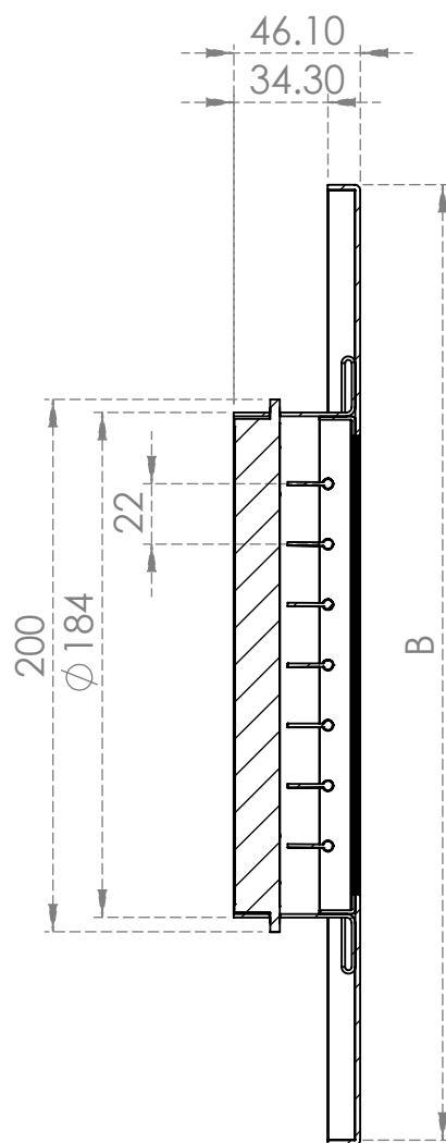
SECTION A-A
