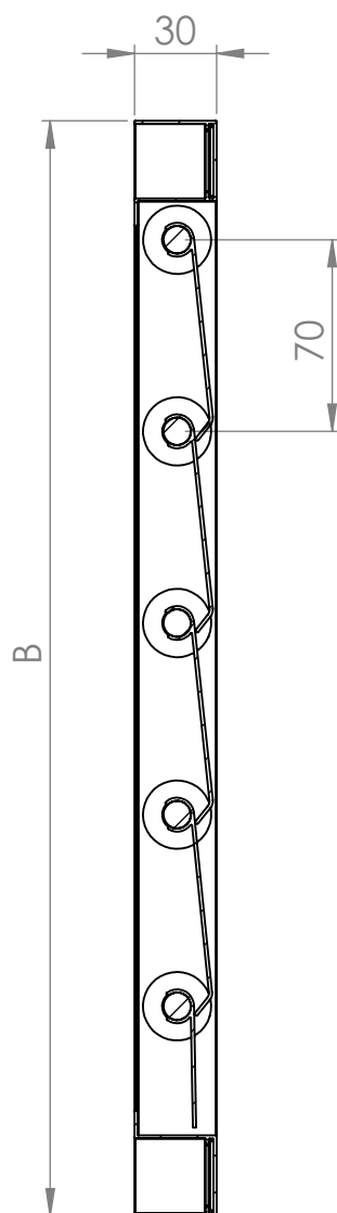
SECTION A-A
