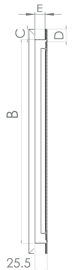
SECTION A-A
