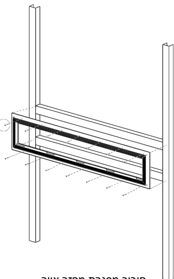
חיבור מסגרת מפזר אוויר ע"י בורג קודח לקונסטרוקציה גבס
