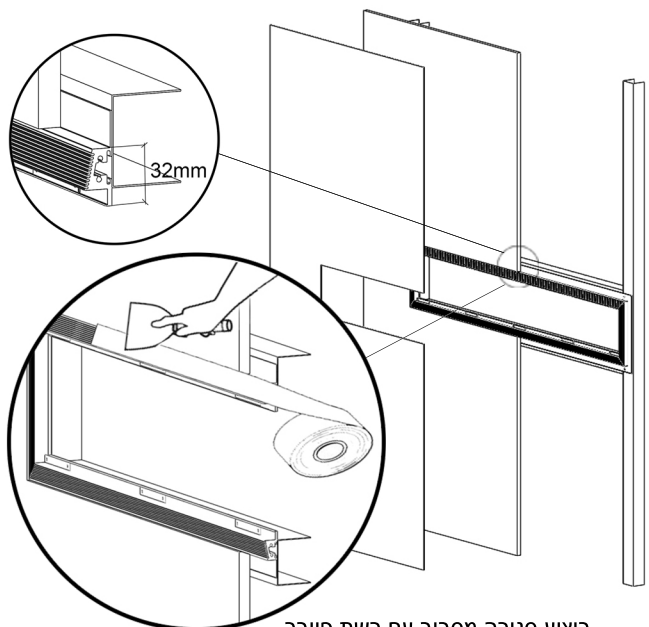
ביצוע סגירה מסביב עם רשת פייבר 3 שכבות שפכטל לגבס
