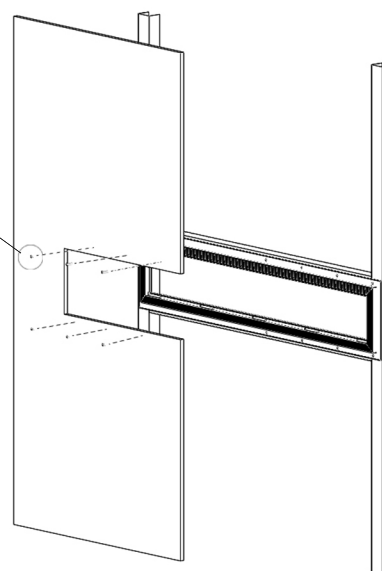
ביצוע מסגרת לפי גודל המפזר בגבס וחיבור פלטת הגבס עם ברגים
