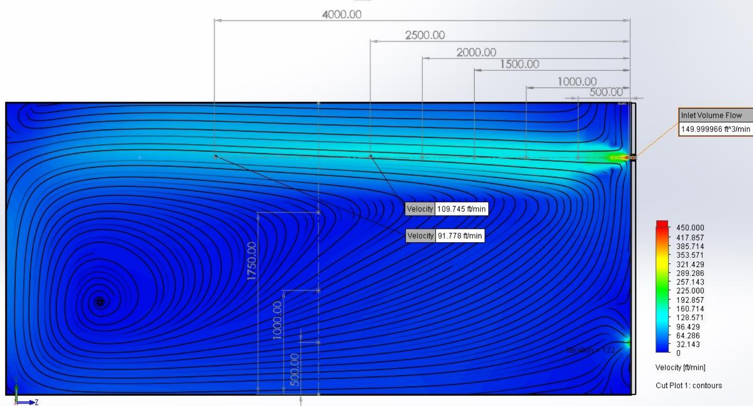
*הדמיית פיזור אויר קירי זריקה ישרה (30mm), בחלל בטמפרטורה אחידה, כניסה של 150 CFM.
