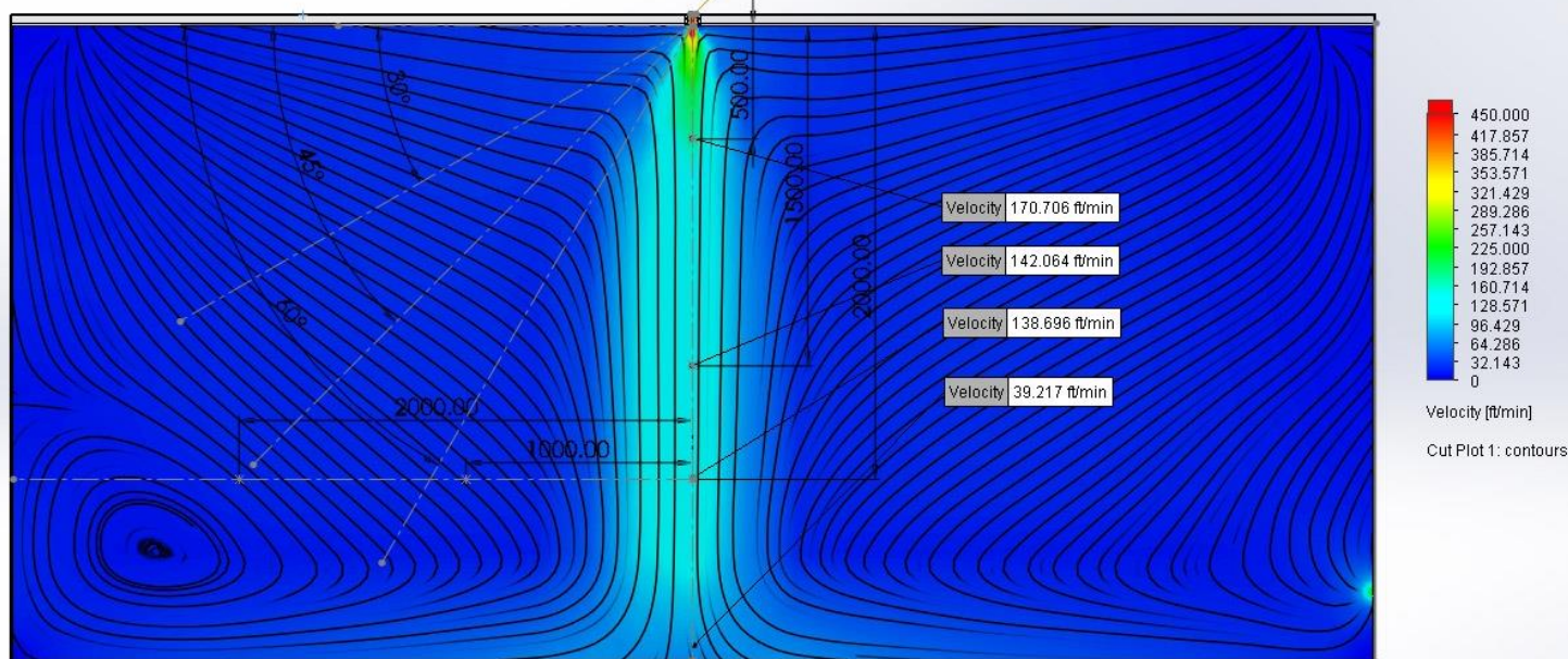
*הדמיית פיזור אויר תקרתי זריקה ישרה (30mm), בחלל בטמפרטורה אחידה, כניסה של 150 CFM.
