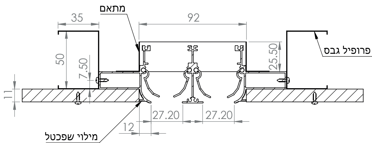
SECTION A-A SCALE 1 : 2
