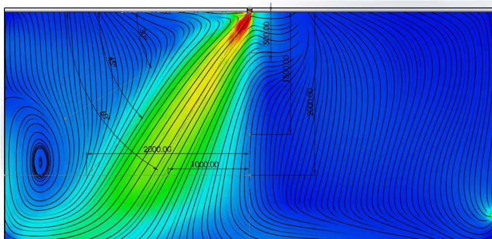
*הדמיית פיזור אויר תקרתי, זריקה בזווית בחלל בטמפרטורה אחידה.
